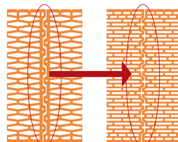
tradiční řešení spoje cihel Porotherm 44
